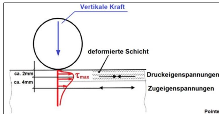
Abbildung 6: Spannungszustand unter der Rad- und Schienenoberfläche
